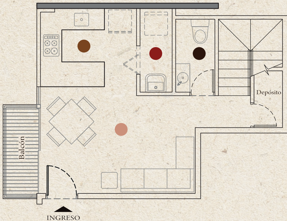
Planta Baja
